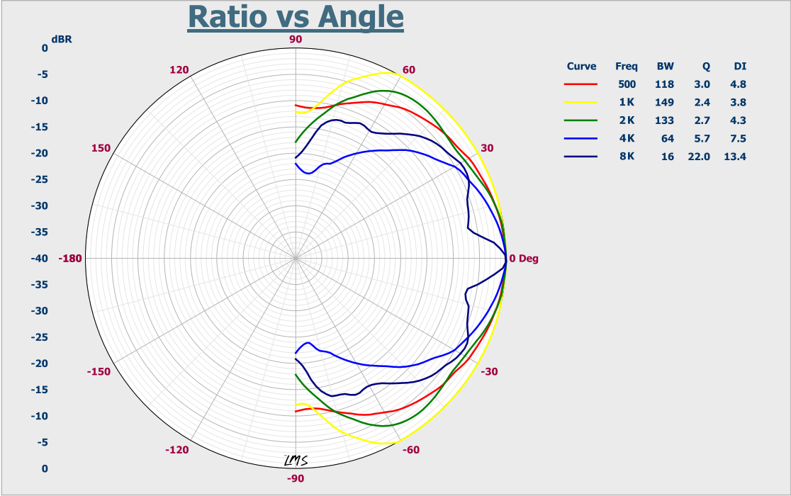
Круговая диаграмма направленности громкоговорителя LPA-6C EVA
